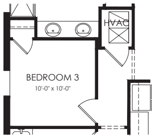
Bedroom 3
